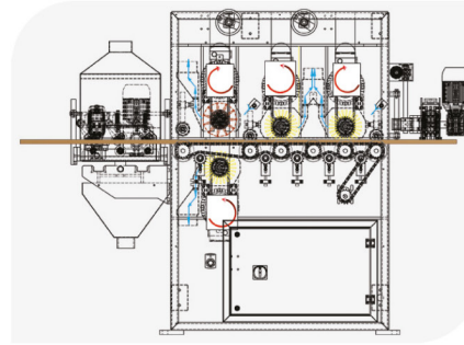
Makineye Ait Teknik Çizim Technical Drawing for the Machine
