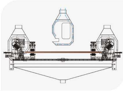
Panelin Alt Kenarlarındaki Çapakları Kırma Freze Modülleri The Milling Models for Breaking Burr in the Lower Edge of Panel
