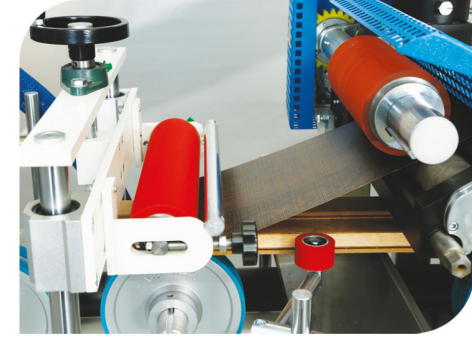
Tutkallanmış Malzemeyi Kesişim Noktasında Hizalayan Baskı Merdanesi The Press Roll is Align Glued Material in Intersection Point
