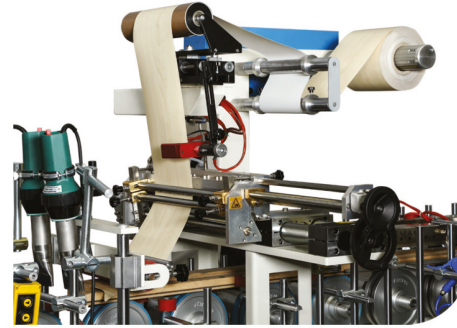
Kusursuz Folyo Yonerdirmeleri için Özel Tasarlanmış Kenar Kontrol Sistemi Special Foil Edge Control System for Perfect Routing
