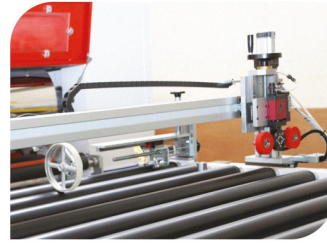
Panelin Boy Ölçüsünü Belirleyen Enkoder Teker The Encoder Wheel for Determining of Size Measure
